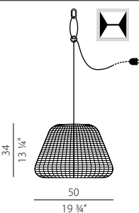
Versione con O-Ring IP65 O-Ring version IP65
