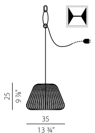
Versione con O-Ring IP65 O-Ring version IP65
