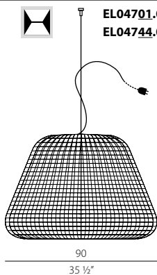
Versione con spina IP65 Version plug IP65
